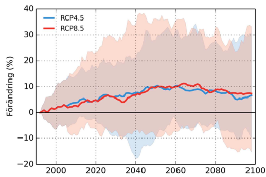
Oxundaån
