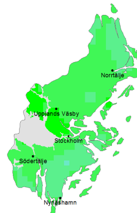
Beräknat 2069-2098
