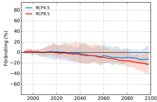
Oxundaån
