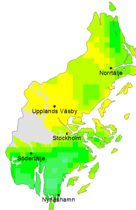
Beräknat 2021-2050
