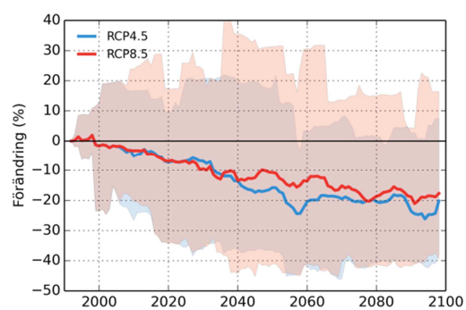
Norrtäljeån
