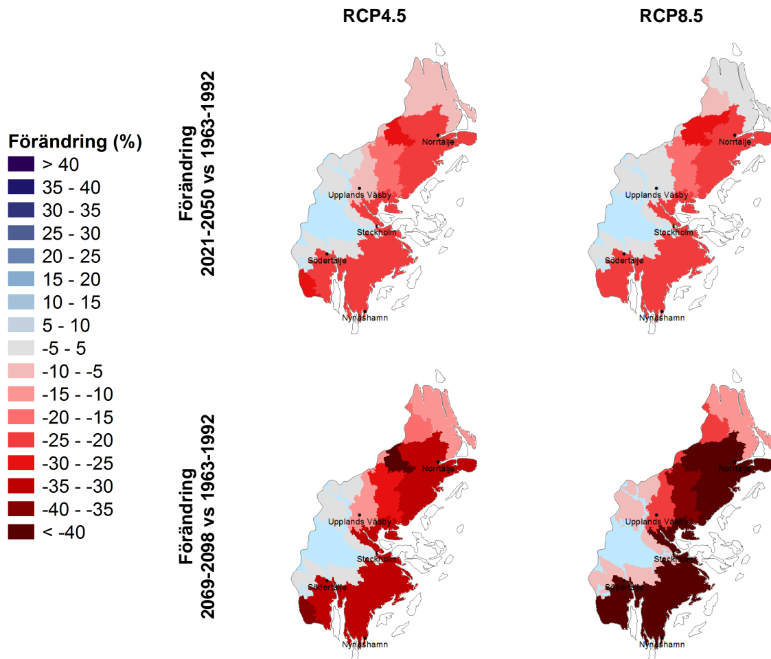
Norrtäljeån
