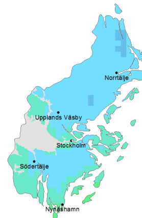
Beräknat 2069-2098
