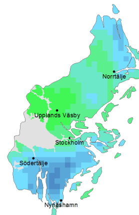
Beräknat 2069-2098
