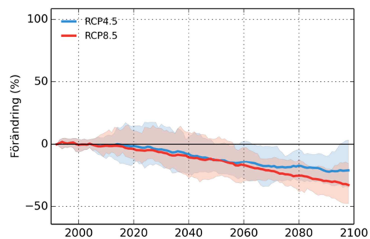
Tyresån
