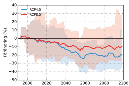
Tyresån
