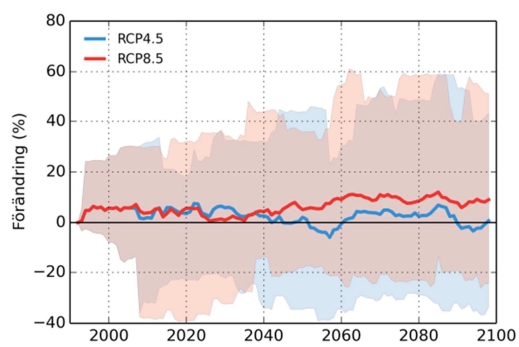
Oxundaån
