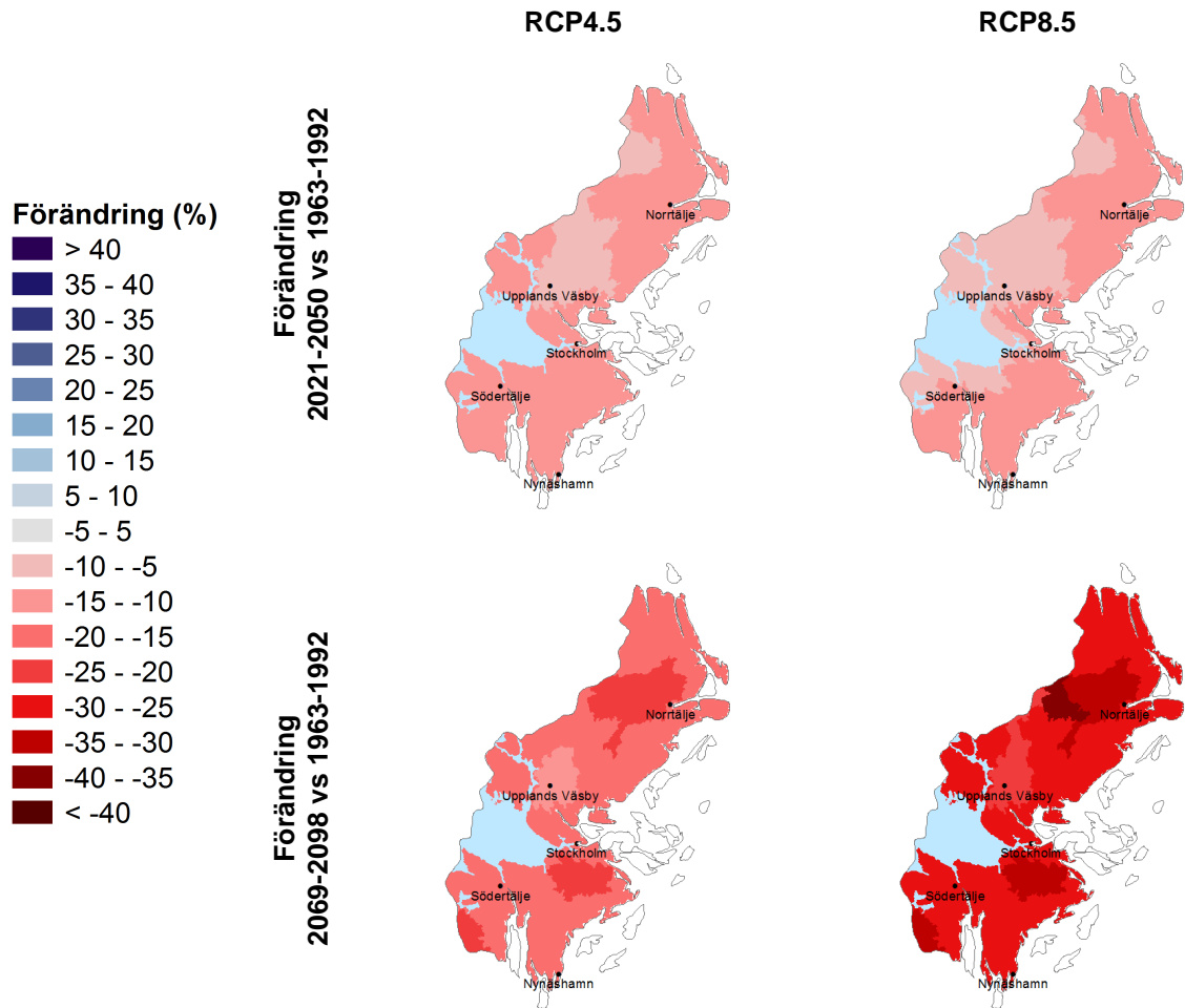
Norrtäljeån
